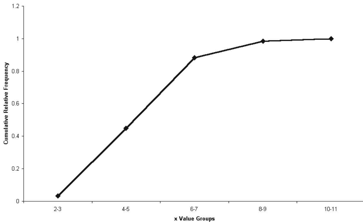
Ogive
